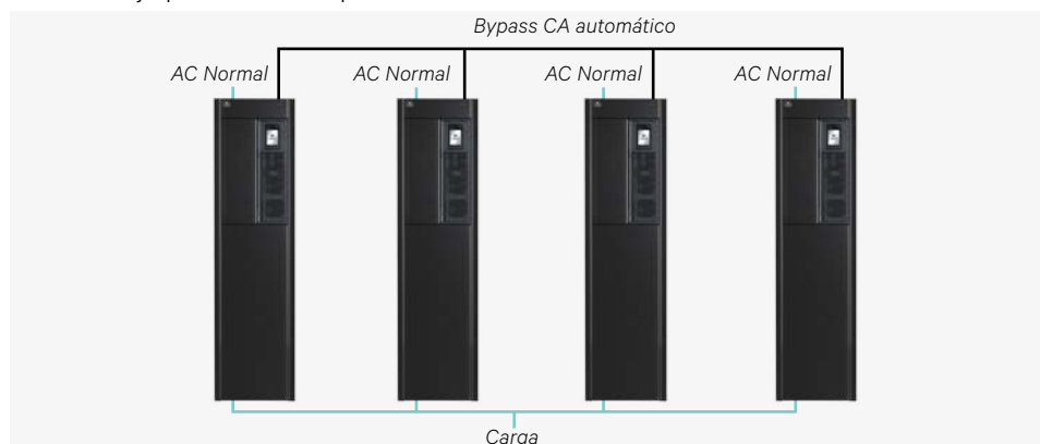
Liebert EXS - Configuração em paralelo
