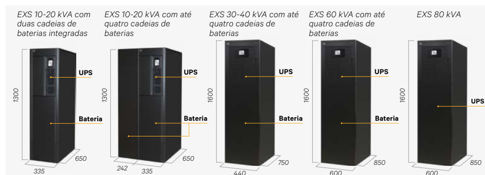
Arquitetura do Liebert EXS
